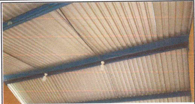
Foto 2: se observa estructura del lado interno.
